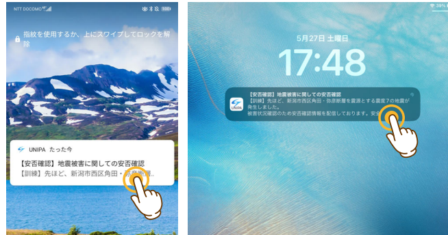
<Android>
